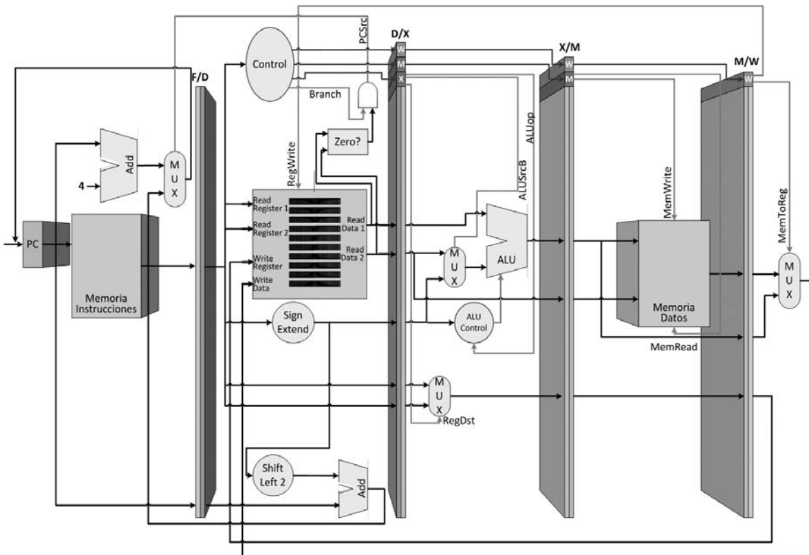
Ruta de datos del nanoMIPS modificada para que las paradas por riesgo de control sean de un ciclo en lugar de tres.
