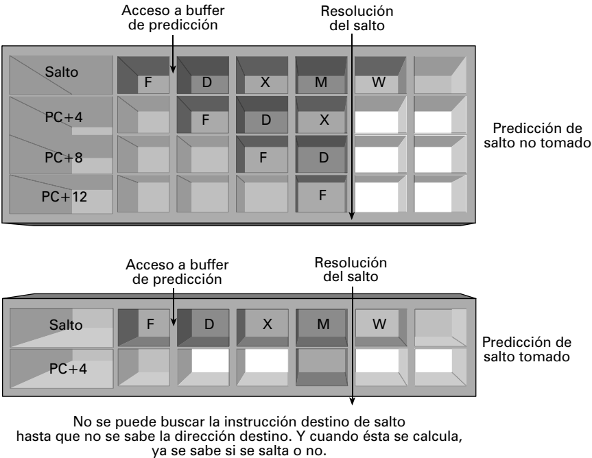
Utilización de un buffer de predicción de saltos en el nanoMIPS que resuelve los saltos en la etapa M.
