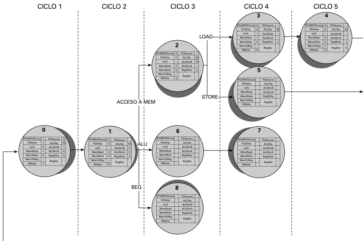
Diseño de la unidad de control para el nanoMIPS multiciclo como máquina de estados.
